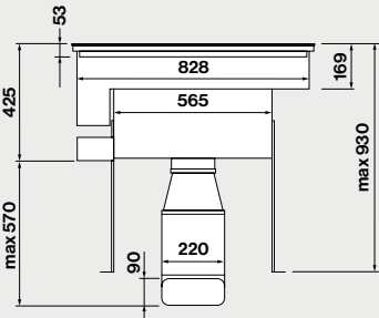
Seitenansicht mit Motor in Frontstellung (Wandmontage)
