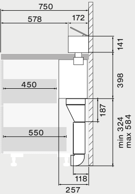
Installationsbeispiel Wand Installation Seitenansicht mit Motor zur Front bei 75 cm Arbeitsplatten Tiefe
