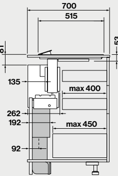
Seitenansicht mit Motor in Heckstellung mit Silence Kit 103076
