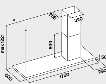
Schacht Rechts
