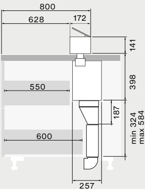
Insel Installation Seitenansicht mit Motor nach hinten
