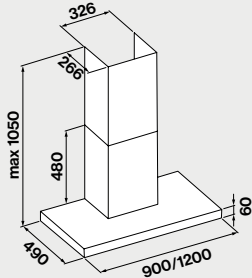
Wand
