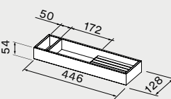
Messerfach 102903
