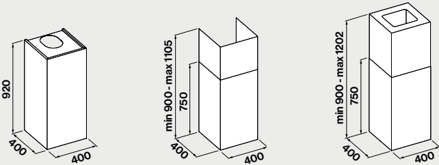
Wand Schwarz / Weiß Wand (Teleskop) Edelstahl Insel
