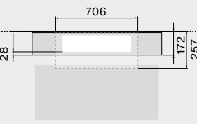
Draufsicht mit Motor zur Front
