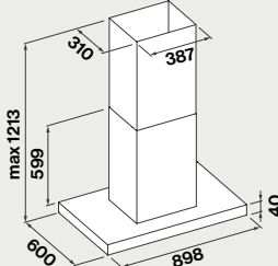
Insel
