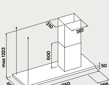
Schacht Rechts
