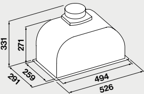
Ausschnitt 50 cm: 262 x 506 mm
