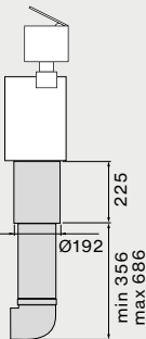
Silence Kit 103076
