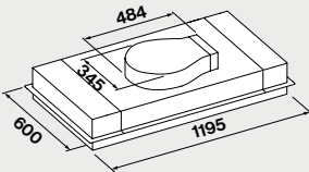
Flacher Motor (nur auf der Haube)
