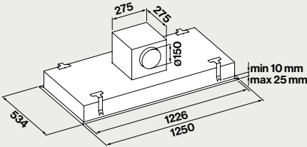
Zwischenkammergebläse / Würfel auf der Haube installiert
