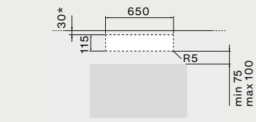
Ausschnitt
