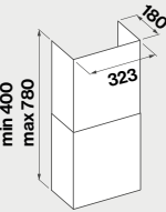
Schacht optional
