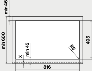
Ausschnittmaß
