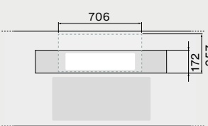
Draufsicht mit Motor nach hinten (Installation mit Motor in hinterer Position nur bei Insel Installation möglich)
