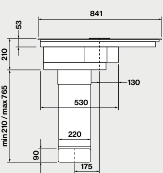
Frontansicht
