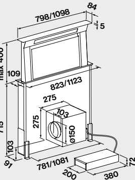
Ablufthaube mit Würfelmotor 950 m³/h
