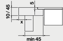
Flächenbündig
