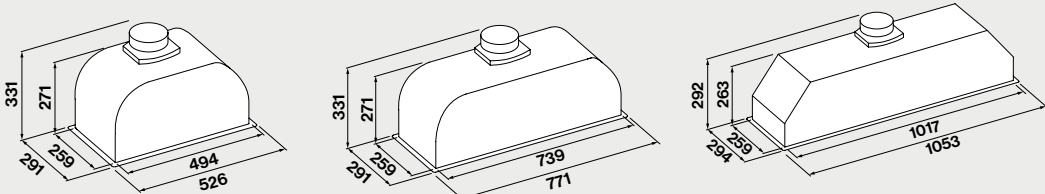
Ausschnitt 50 cm: 262 x 506 mm 70 cm: 262 x 751 mm 105 cm: 262 x 1029 mm
