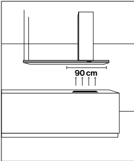
Absaugbereich 90 cm unter dem Schacht
