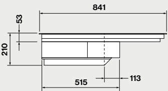
Frontansicht
