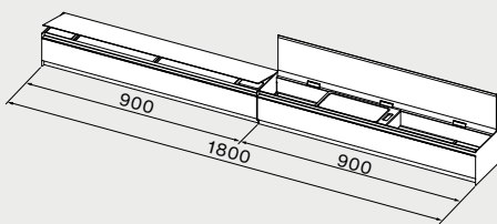
Planungsbeispiel Dunstabzug 90 cm + Ablagemodul 90 cm 102896 + 102898
